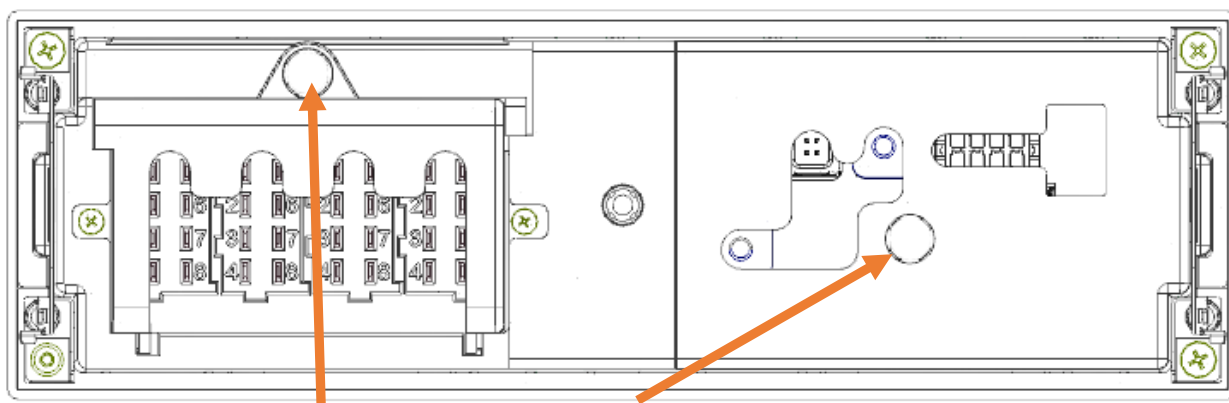
Пластиковая пломба с оттиском номера клейма мастерской
