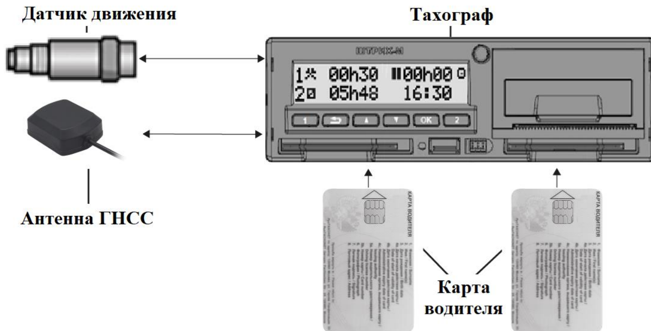
Рисунок 1 – Обзор системы
